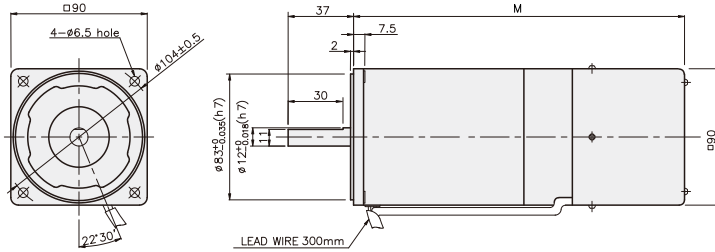
치수도표
