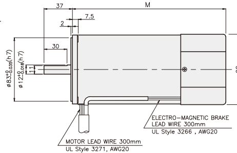
치수도표
