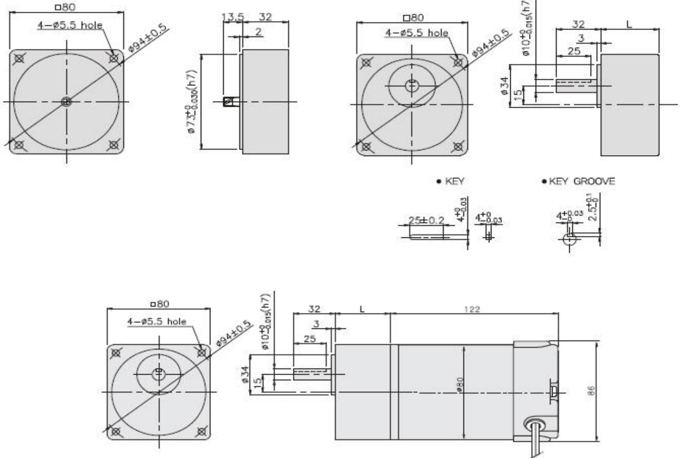
치수도표
